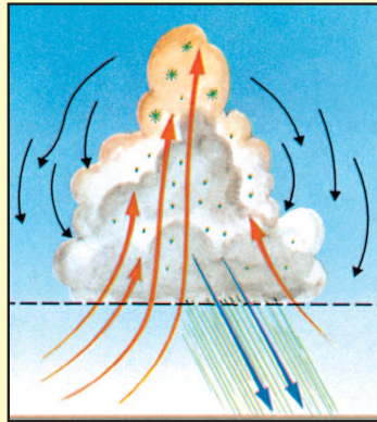
Figuur 20: 'n Cumunolimbus wolk. Hierdie skets dui die opwaartse lugstroming aan. Wanneer die wolk te hoog en swaar word, vind daar 'n neerslag plaas. (Weather and Climate, Bodin, bl.123)
