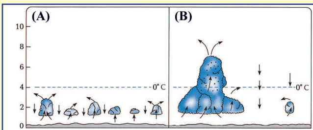
Figuur 19: Water druppels word aangedui deur *
