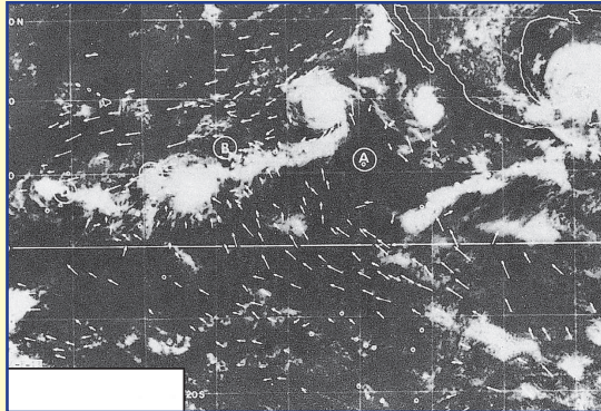
Figuur 17: Hierdie satelliet foto wys hoe die wolke deur lugstrome aangedryf word en dan akumuleer by punt A en B. Die pyltjies dui die windrigtings aan.
