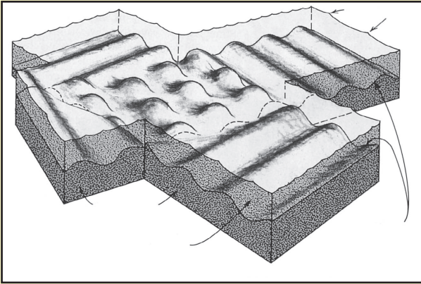
Figuur 16: Interne golwe wat op verskillende digtheidsvlakke plaasvind. Hoe dieper die water is, hoe hoër is die digtheid.
